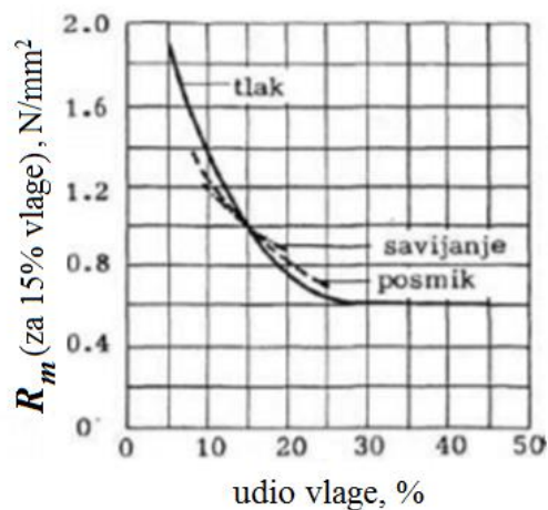
Slika 3.5. Utjecaj vlage na čvrstoću drva [8]
