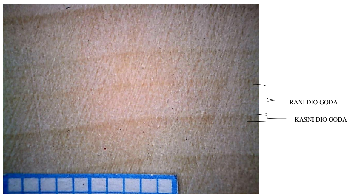
Slika 4.11. Makrostruktura lipe
