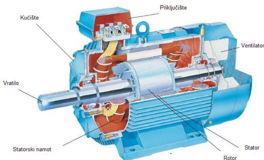
Slika 5.2 Shema asinkronog motora [10]
