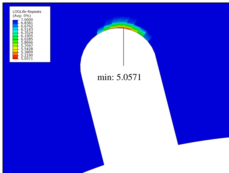
Slika 53. Kritično područje nastanka pukotine kod zupčanika s tankim vijencem
