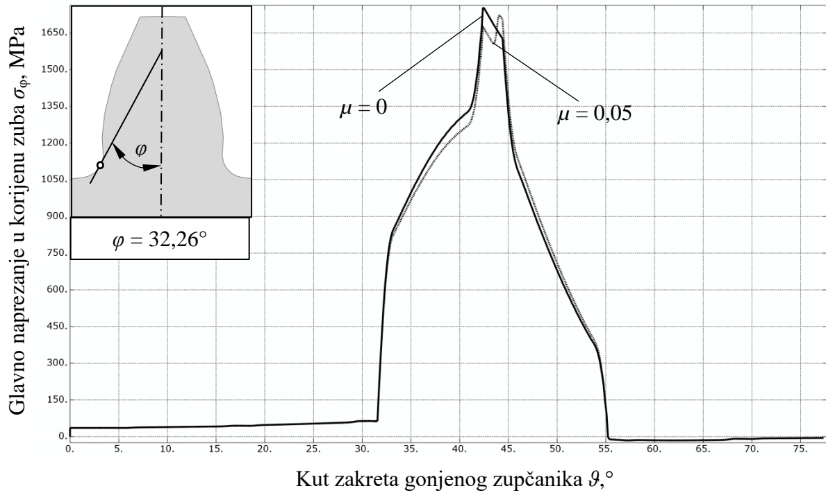
Slika 56. Utjecaj trenja na ciklus napreznja punog zupčanika sa zarezom
