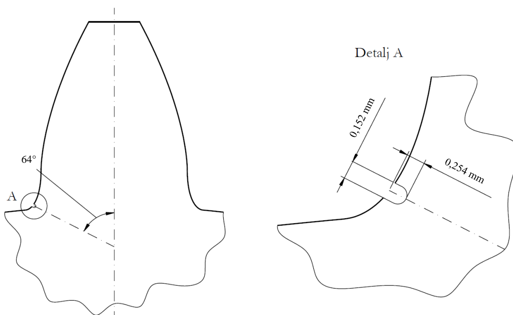
Slika 33. Dimenzije i pozicija zarezalazi na zupčaniku s tankim vijencem [5]
