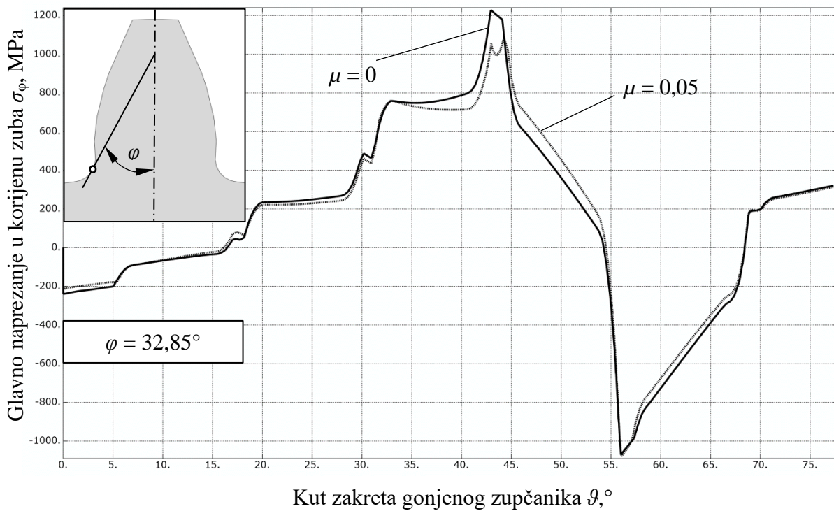
Slika 57. Utjecaj trenja na ciklus napreznja zupčanika s tankim vijencem i zarezom
