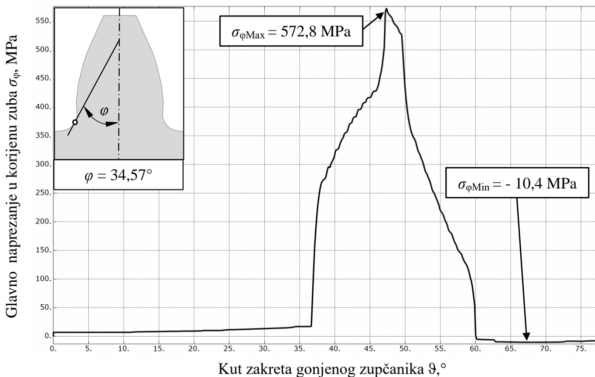
Slika 24. Ciklus napreznja korijena zuba punog zupčanika bez zarezata
