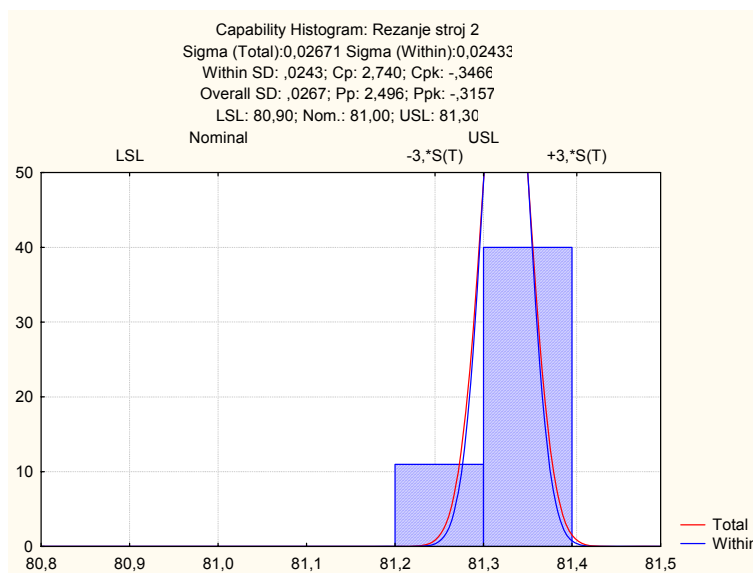
SI. 46. Histogram sposobnosti izmjerenih dužina cijevi nakon eliminacije podataka
