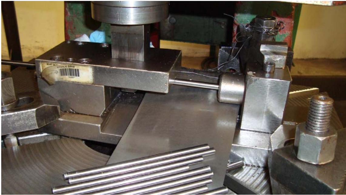
Sl. 17. Odsijecanje šipke
