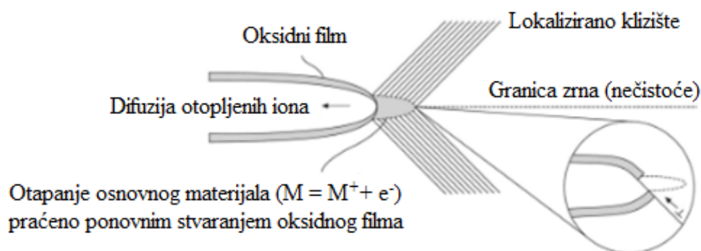
Slika 19: Otapanje osnovnog metala u aktivnom području razaranja [21]
