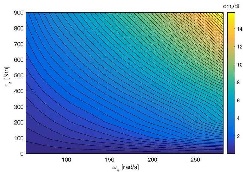
Slika 8. Prikaz mape potrošnje goriva iskazan u g/s
