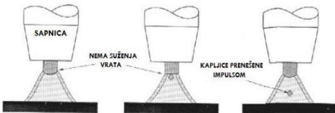
Slika 11. Schematski prikaz prijenosa metala impulsnim lukom [14]
