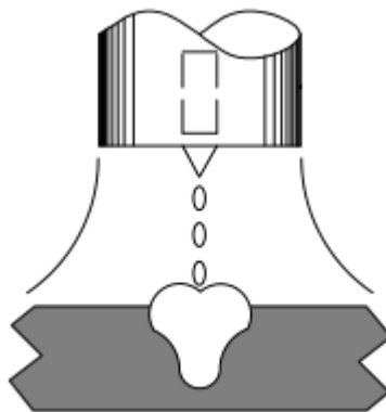
Slika 10. Shematski prikaz prijenosa metala štrcajućim lukom [12]
