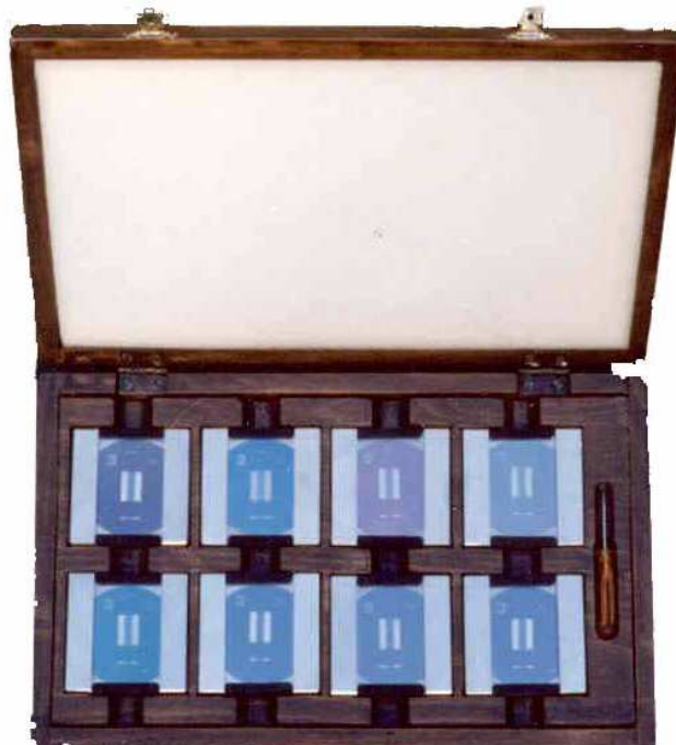
Slika 2.1. Set referentnih etalona hrapavosti LFSB-a.
