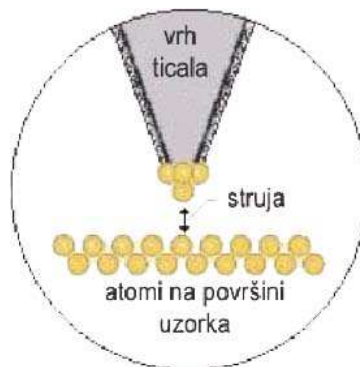
Slika 1.22. Vrh ticala STM-a.
