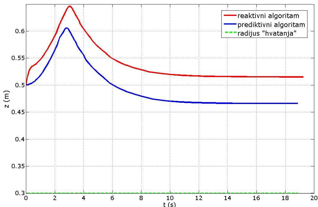
Slika 5.13. Udaljenosti između mobilnih robota za slučaj međusobno okomito orijentiranih mobilnih robota ( \pi/2 ) u početnom položaju, pravocrtnog gibanja prvog mobilnog robota i vremenskog horizonta predikcije T = 1 s
