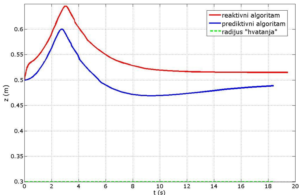
Slika 5.16. Udaljenosti između mobilnih robota za slučaj međusobno okomito orijentiranih mobilnih robota ( \pi/2 ) u početnom položaju, pravocrnog gibanja prvog mobilnog robota i vremenskog horizonta predikcije T = 3 s
