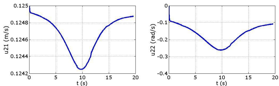
Slika 5.34. Upravljačke varijable drugog mobilnog robota za slučaj međusobno okomito ( \pi/2 ) orijentiranih mobilnih robota u početnom položaju, polukružnog gibanja prvog mobilnog robota i vremenskog horizonta T = 3
