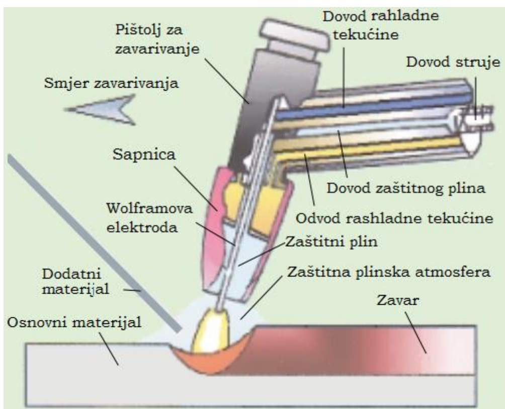
Slika 3. Shematski prikaz TIG postupka zavarivanja [8]
