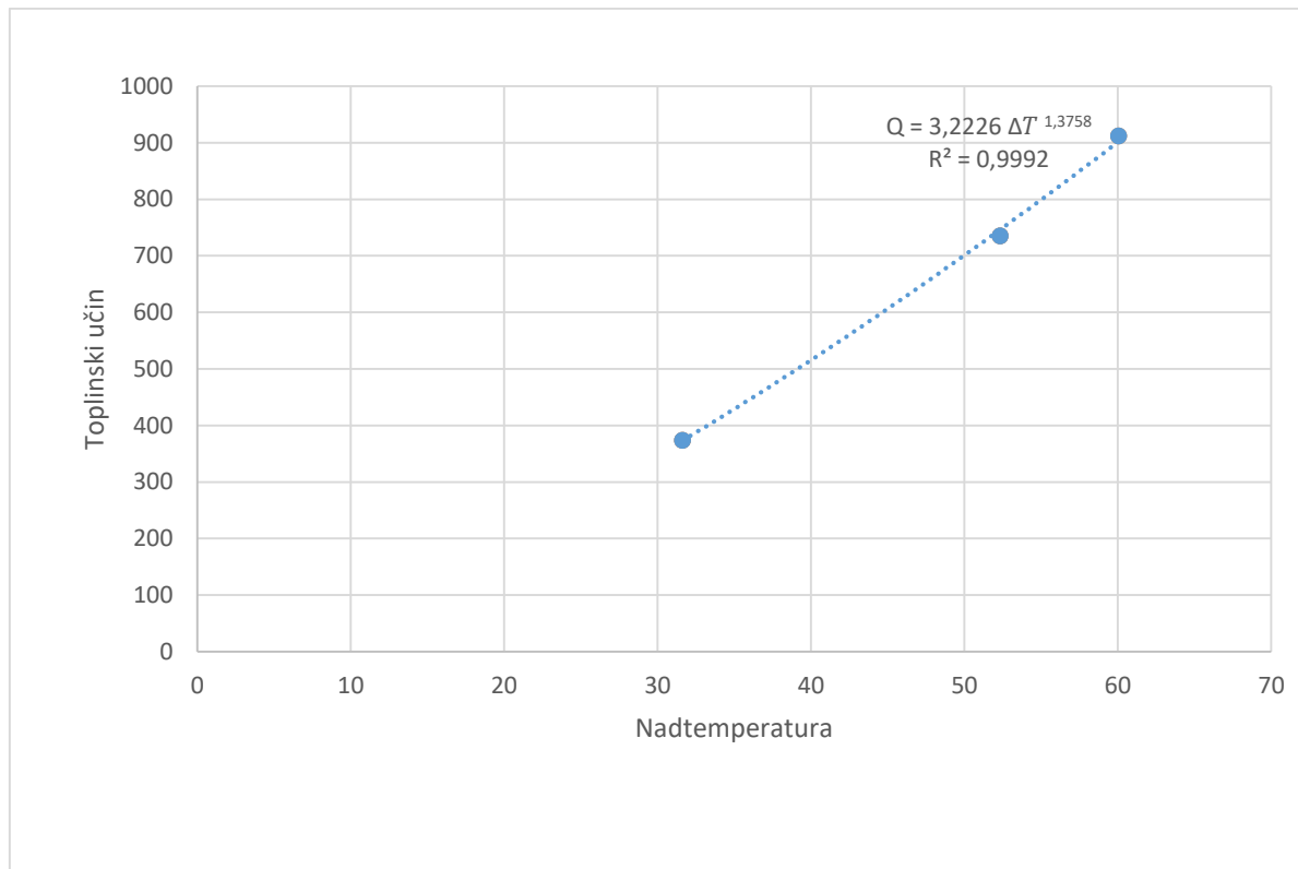
Slika 11. Karakteristična jednađžba konvektora
