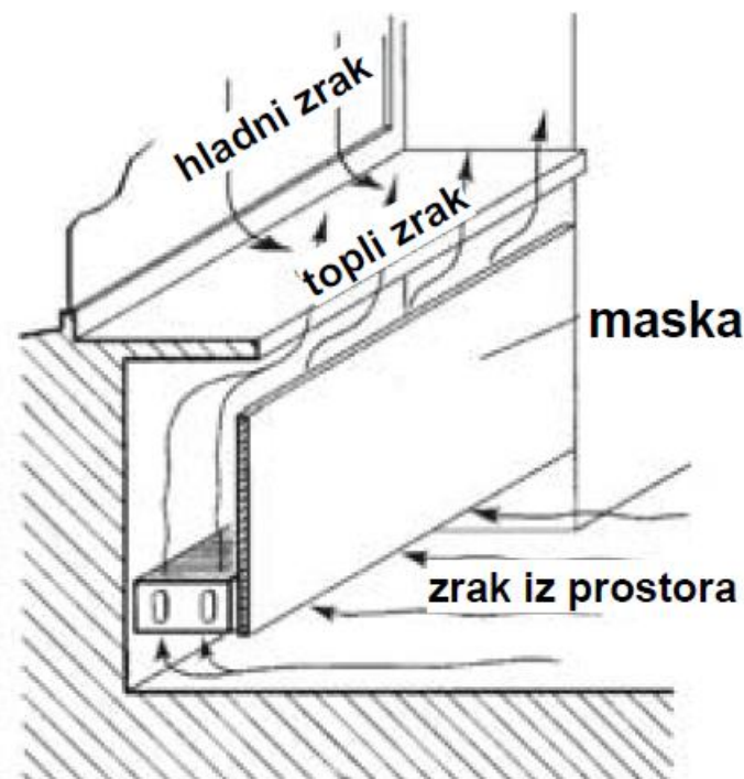
Slika 2. Princip rada konvektora
