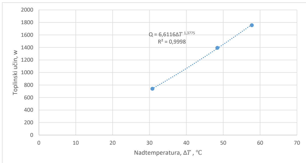
Slika 9. Karakteristična jednadžba radijatora
