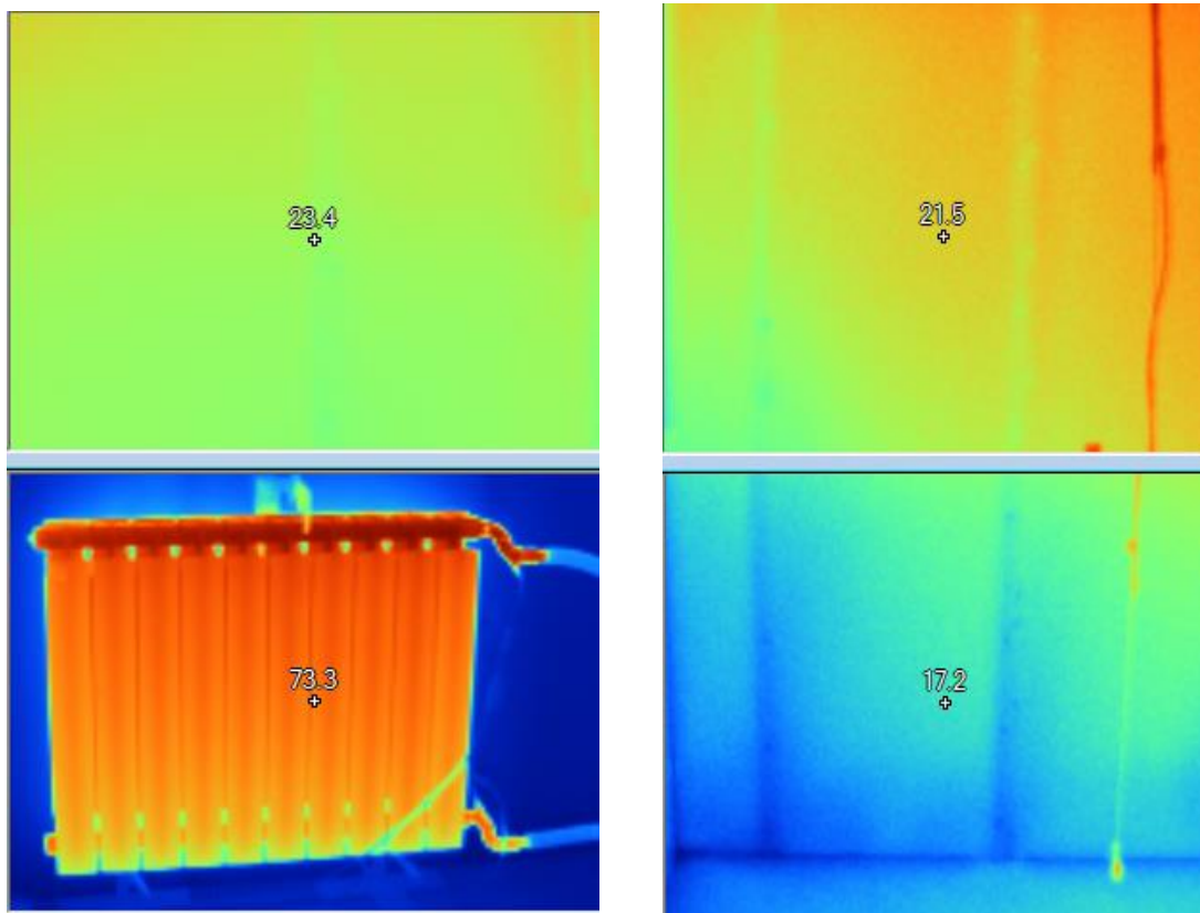
Slika 21. Temperatura radijatora( lijevo) i zida nasuprot radijatoru (desno) za \Delta 60 °C
