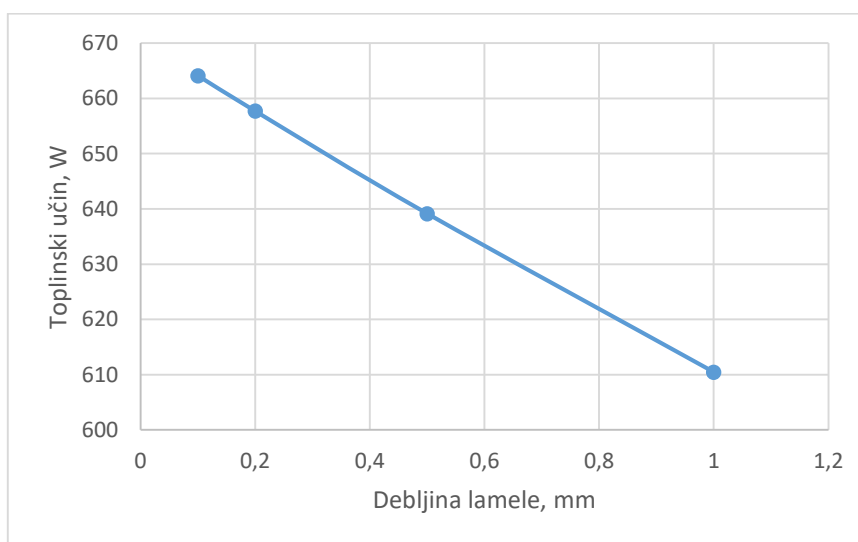
Slika 13. Utjecaj debljine lamele na toplinski učin
