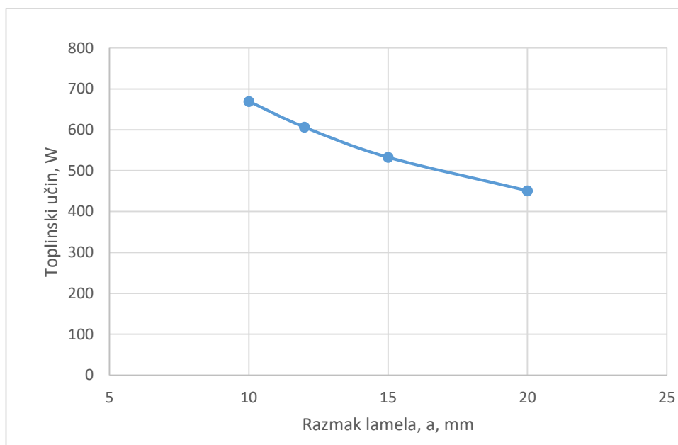
Slika 14. Utjecaj razmaka lamele na toplinski učin
