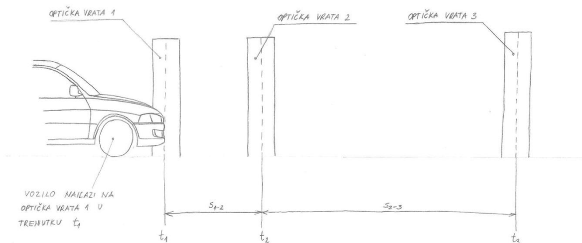
Slika 33. Shematski prikaz postupka mjerenja usporenja vozila pomoću optičkih vrata
