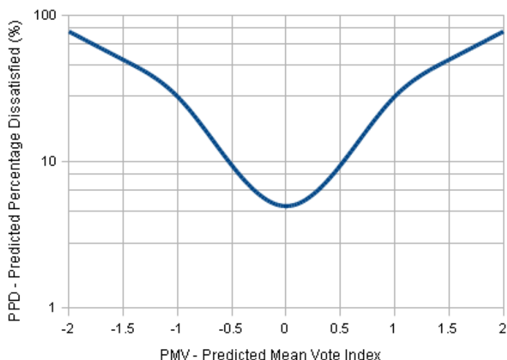
Slika 1.1. Ovisnost PPD i PMV indeksa
