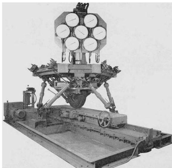
Slika 16. Gough-ova platforma [8]
