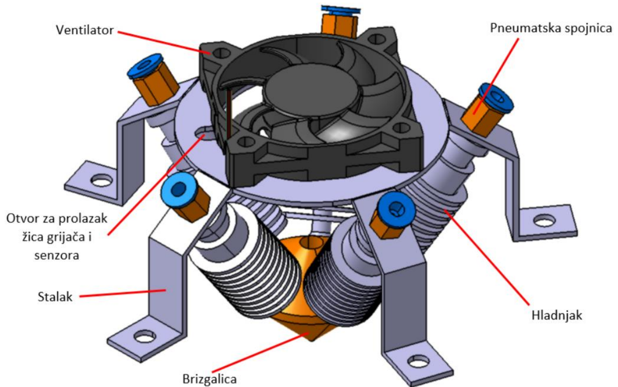
Slika 37. Sustav brizgalice
