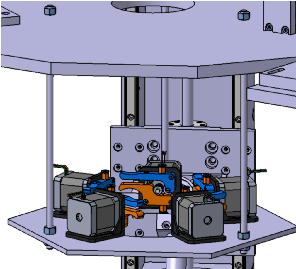
Slika 40. Smještaj ekstrudera
