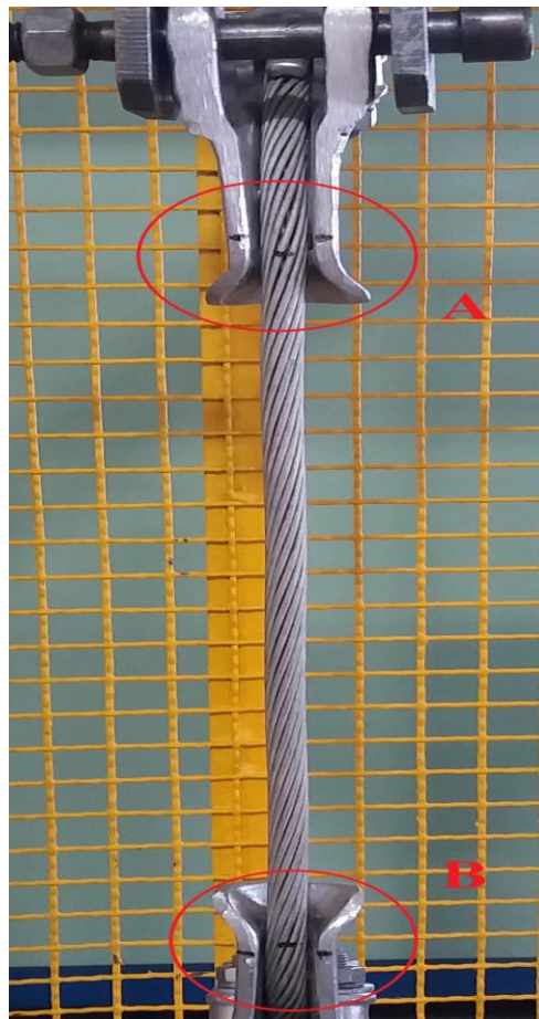
Slika 24. Ispitivanje na kidalici: a) prihvat uzorka na kidalici, b) izvlačenje vodiča iz stezaljke
