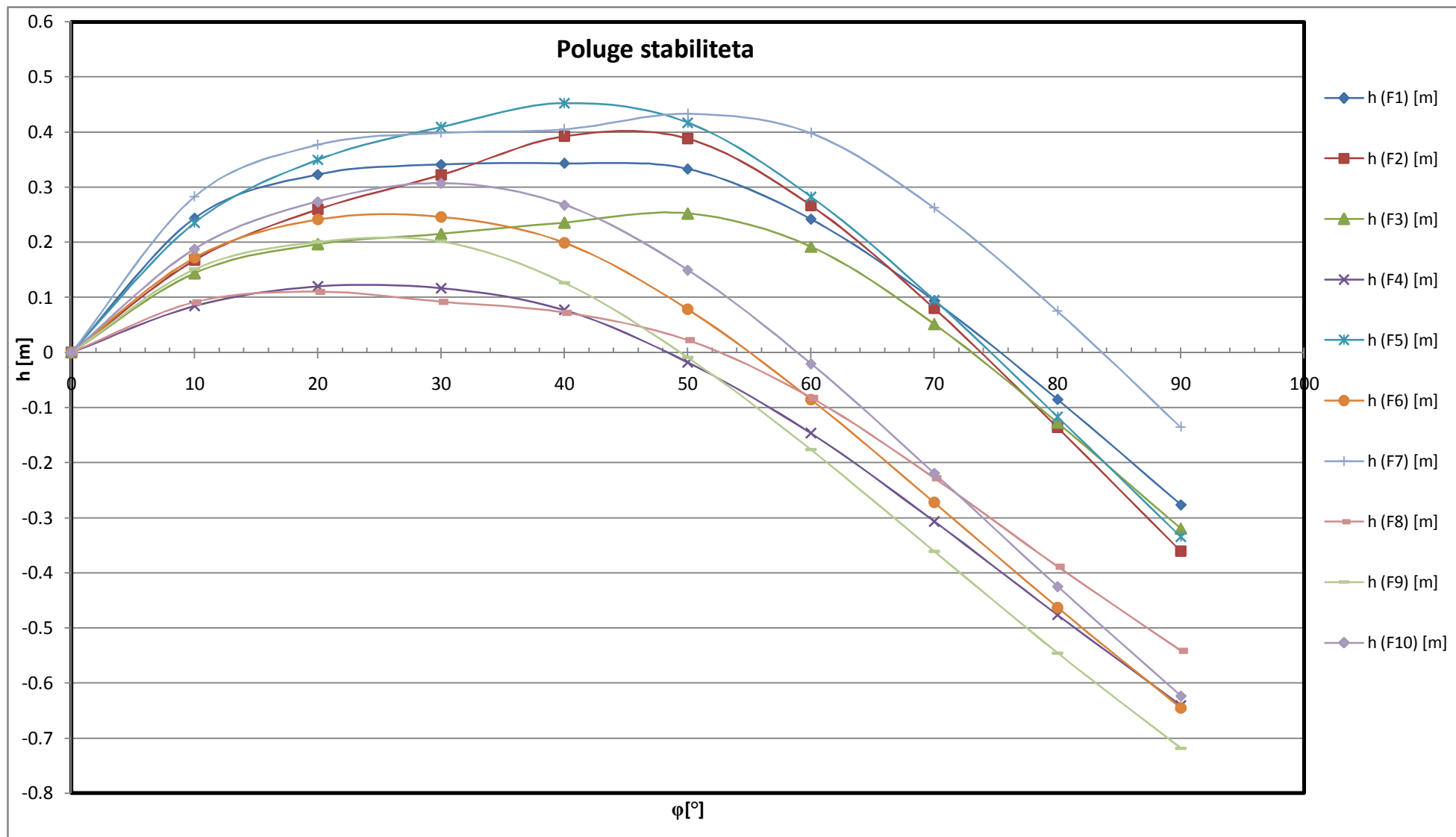
Slika 46-Poluge stabiliteta
