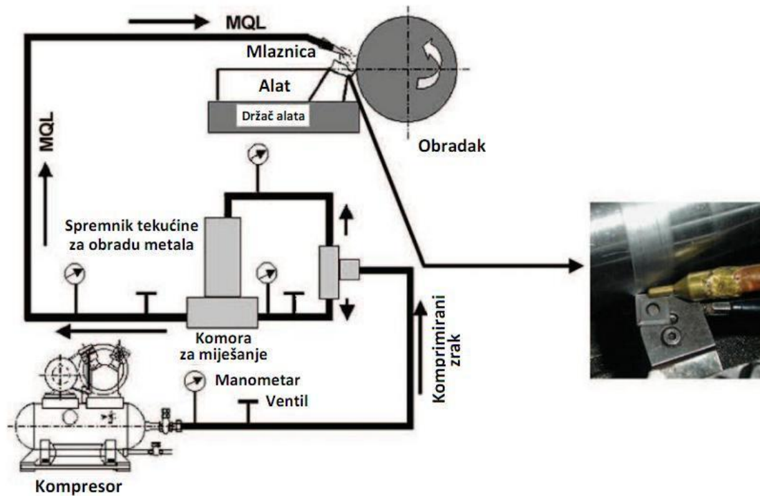
Slika 27. Shematski prikaz eksterne MQL jedinice kod obrade tokarenja [17]
