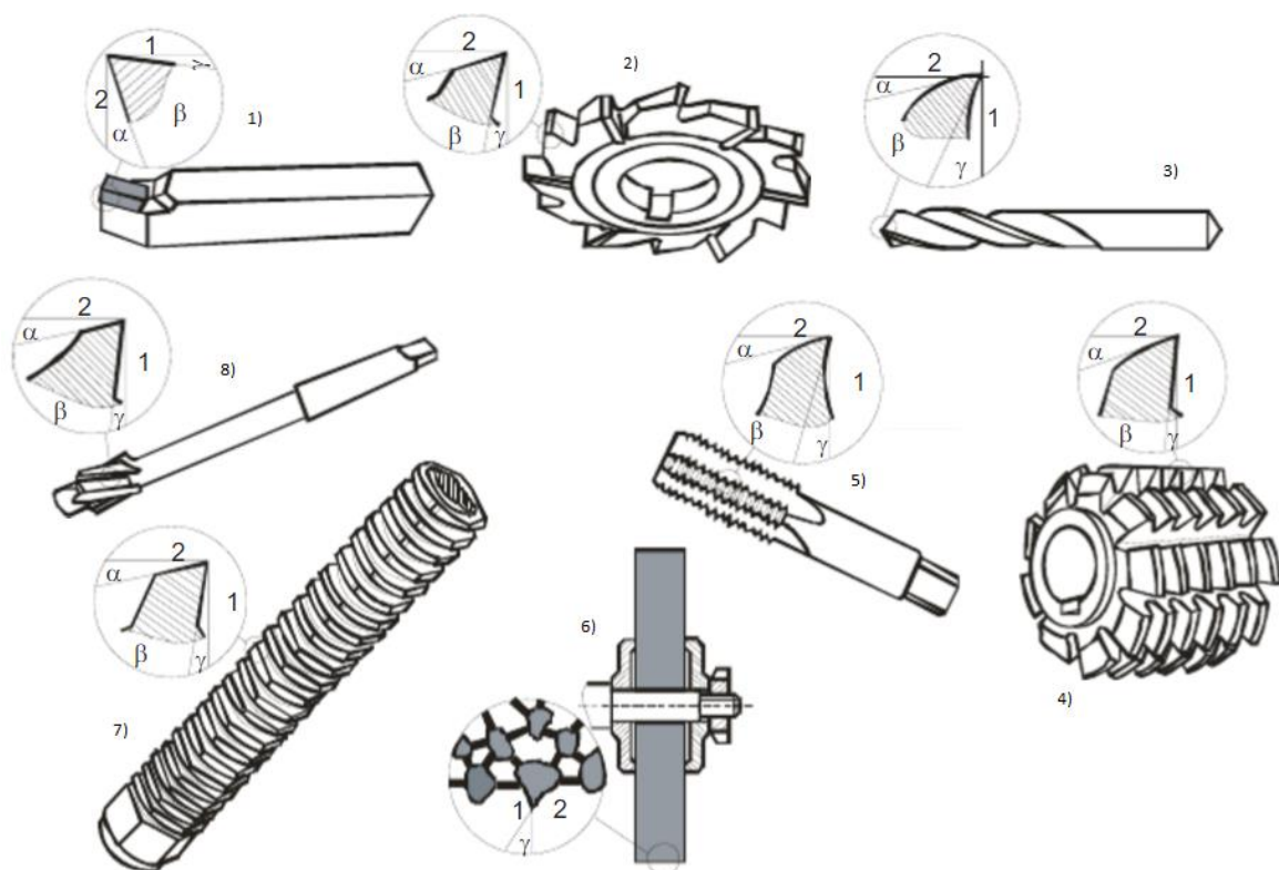
Slika 3. Neki od alata kod obrade odvajanjem čestica [3]
