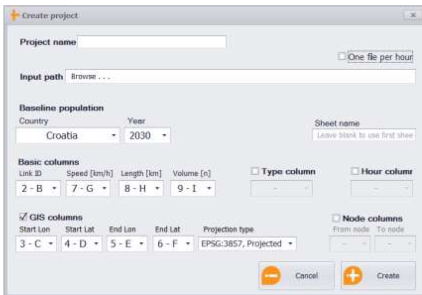
Slika 2.2. Create project
