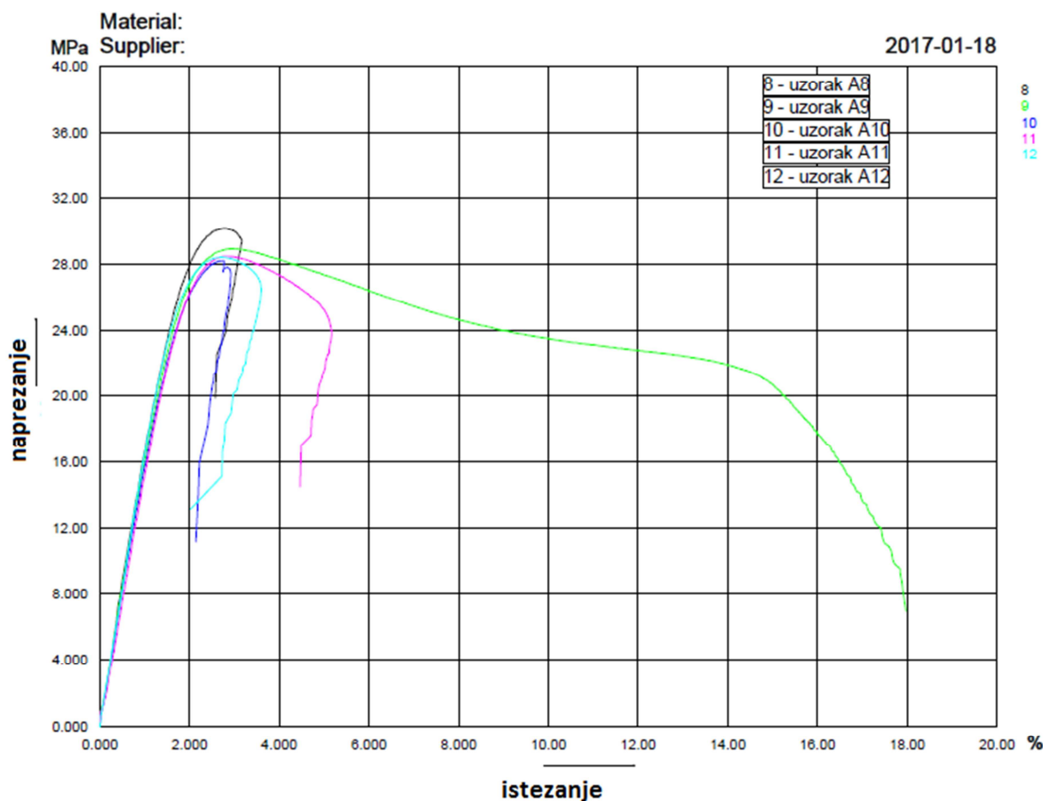
Slika 4.1 Dijagram naprežanje-istežanje za epruvete uzorka A (nepropucana ABS meta)
