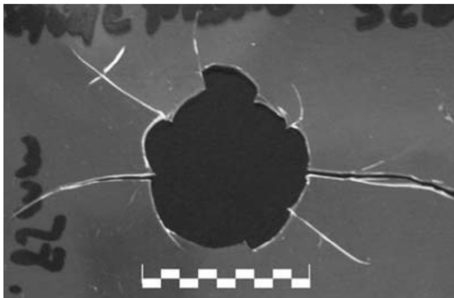
Slika 2.4.3 Izgled krhkog loma EMAA-925 pri -30^{\circ}\text{C} [1]
