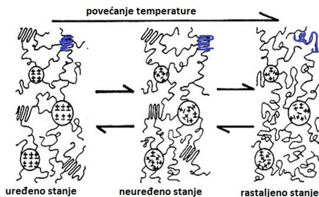
Slika 2.5 Prikaz promjene mikrostrukture za vrijeme procesa zagrijavanja/hlađenja [1]
