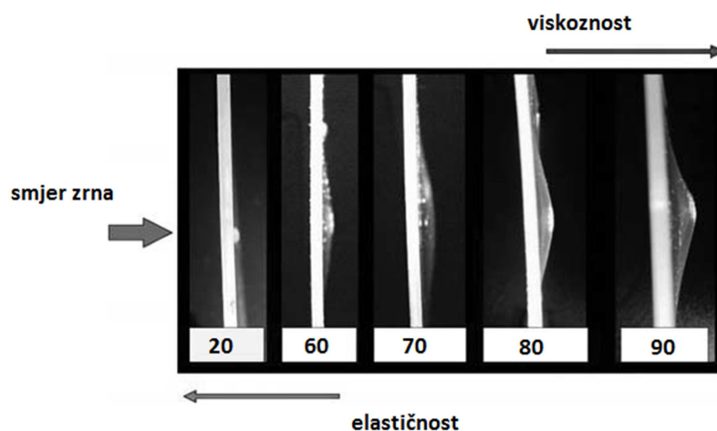
Slika 2.4.2 Utjecaj okolišne temperature na ponašanje ispitnog tijela pri propucavanju [1]
