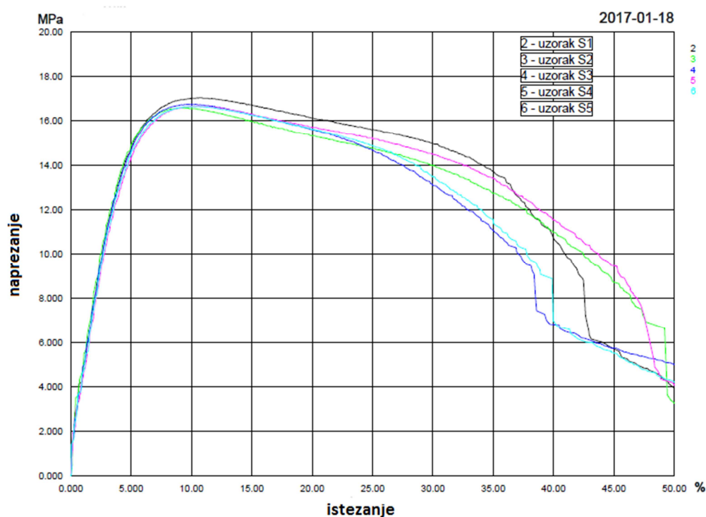
Slika 4.3 Dijagram naprežanje-istezanje za epruvete uzorka S (Surlyn 8940, prostrjeljen s 5,56)
