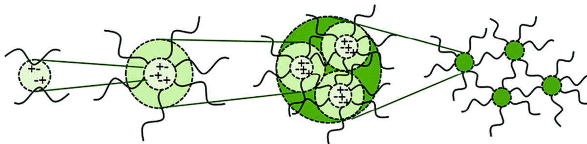
Slika 2.3 Struktura ionomera [1]
