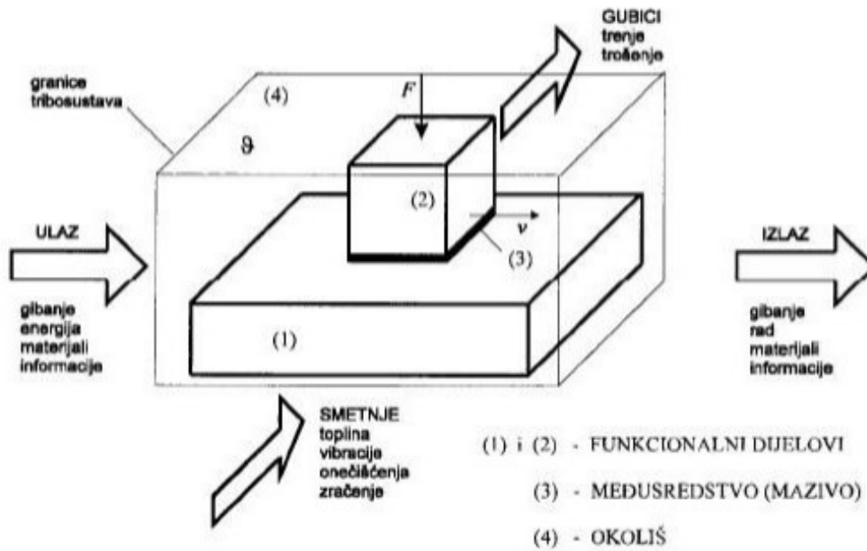
Slika 6. Osnovni tribosustav [11]
