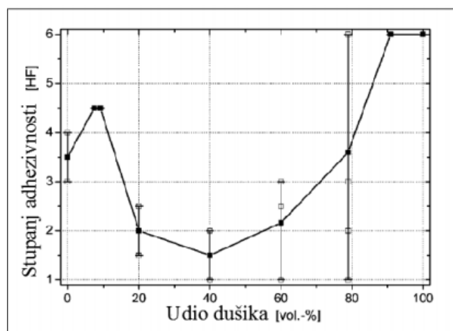
Slika 2.10. Stupanj adhezivnosti TiN prevlake na alatnom čeliku za hladni u ovisnosti o omjeru N 2 /H 2 [11]
