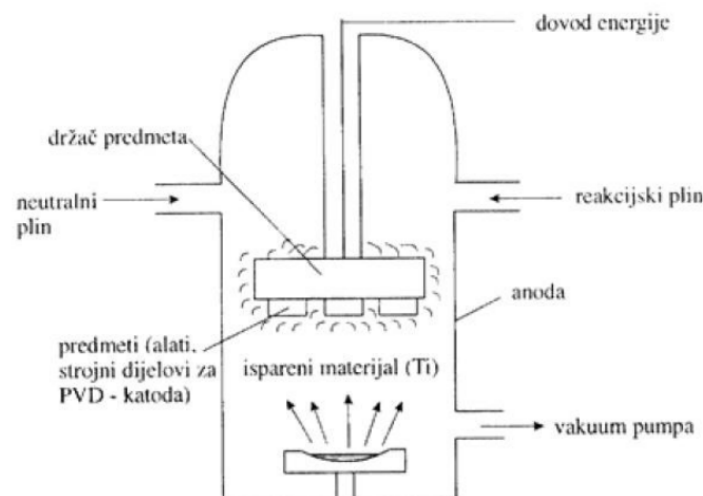
Slika 2.2. Shema uređaja za PVD postupak [3]
