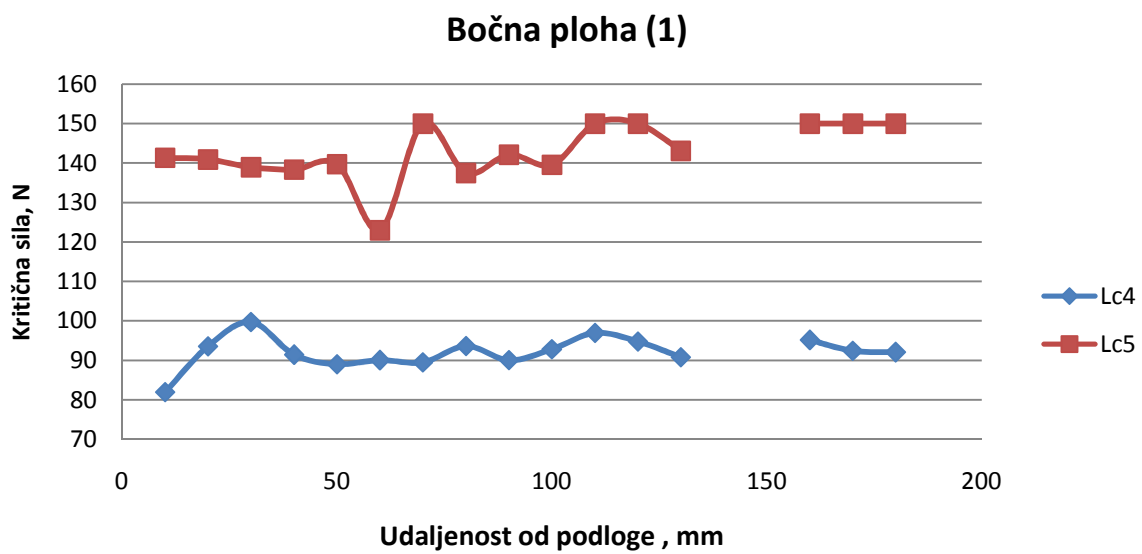
Slika 4.6. Ovisnost kritičnih sila L_{c4} i L_{c5} o udaljenosti od podloge za bočnu plohu uzorka
