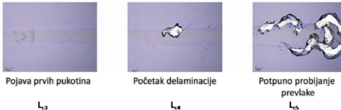
Slika 3.3. Karakteristični događaji i kritične sile ispitivanja prionjivosti brazdanjem [14]
