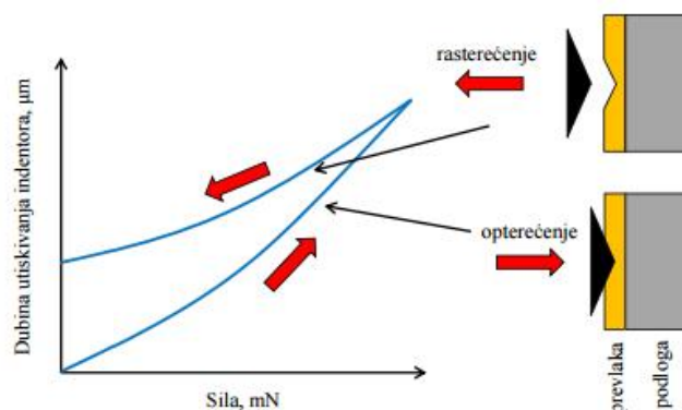
Slika 3.1. Način mjerenja tvrdoće tankih tvrdih prevlaka [14]
