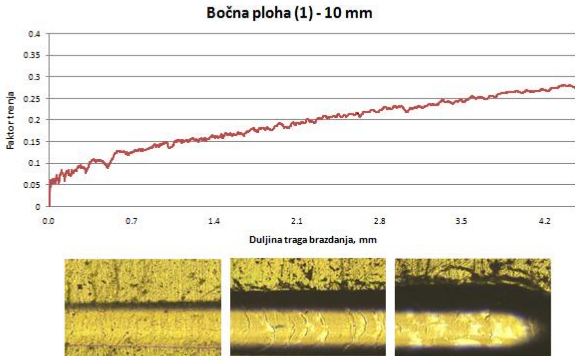
Slika 4.19. Faktor trenja za bočnu plohu uzorka na visini od 10 mm
