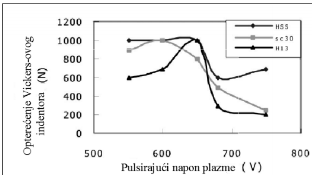
Slika 2.11. Adhezivnost TiN prevlake na različitim pulsirajućim naponima plazme [12]
