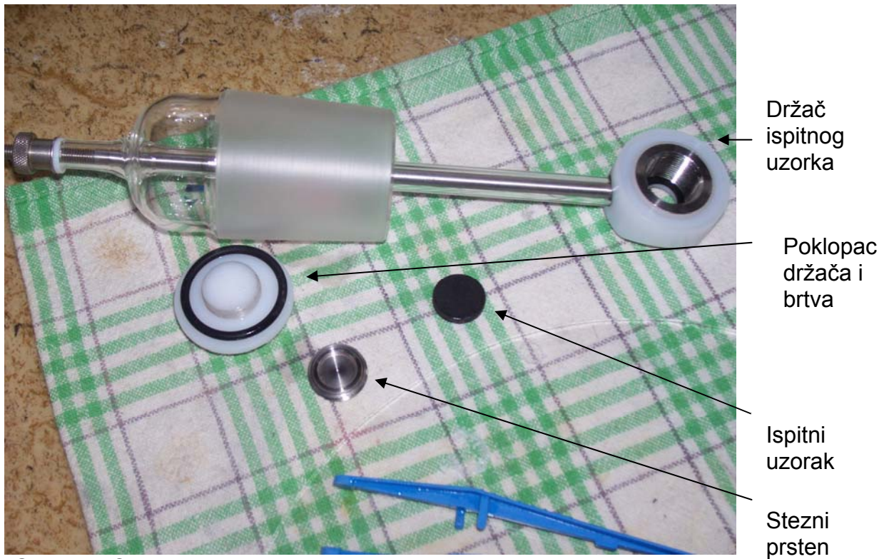
Slika 39. Sastavni dijelovi radne elektrode za ispitivanje elektrokemijske korozije
