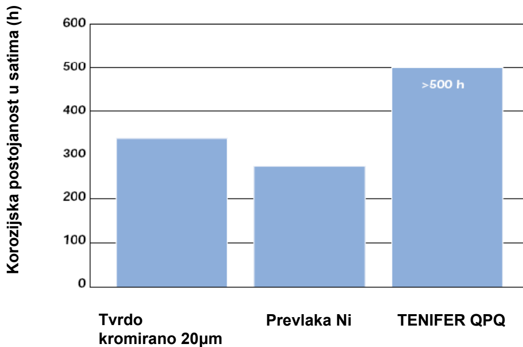
Slika 27: Korozivna otpornost u slanoj magli po DIN 50021 galvaniski nanošenih slojeva u odnosu na sloj dobiven postupkom TENIFER QPQ [ 12 ]
