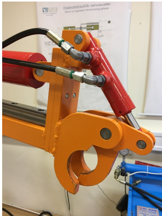
Slika 13. Zatvorena prihvatnica
