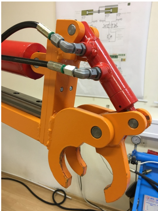
Slika 12. Otvorena prihvatnica
