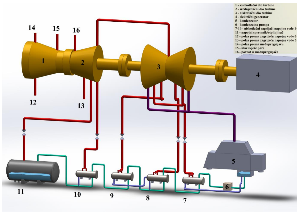
Slika 15. Prikaz dijela postrojenja relevantnog za kondenzat stop
