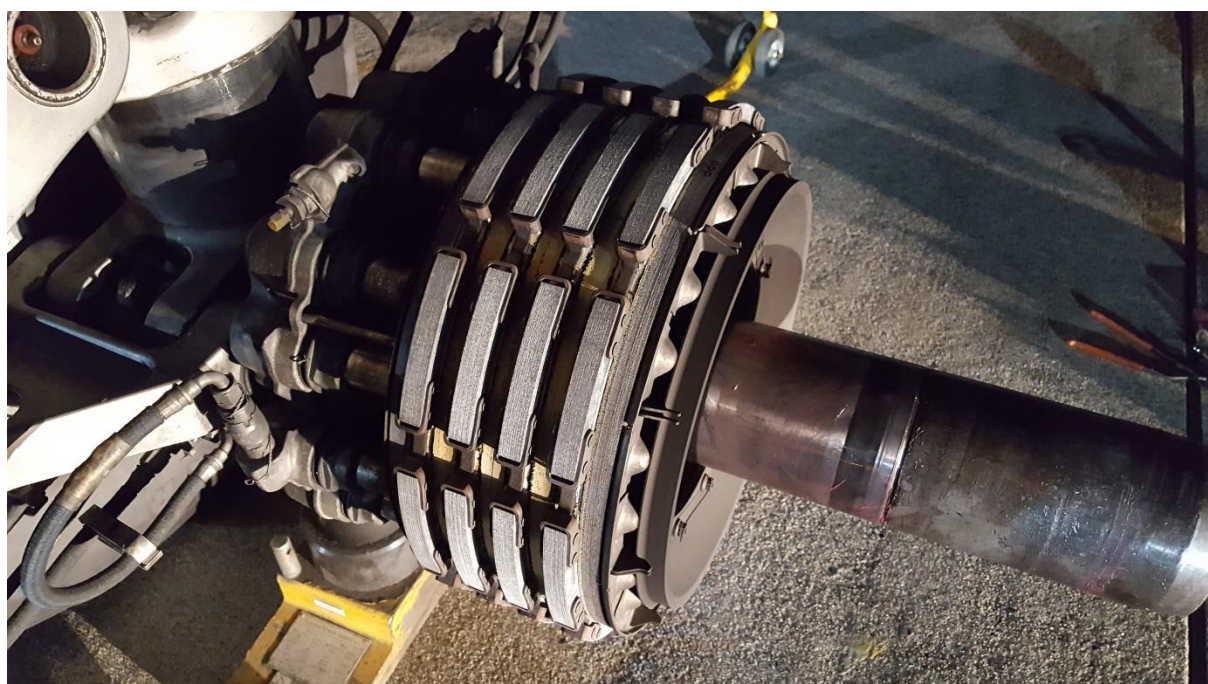
Slika 16. Kočnica zrakoplova
