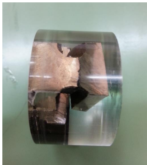
Slika 89. Napuknuće uzorka diska
