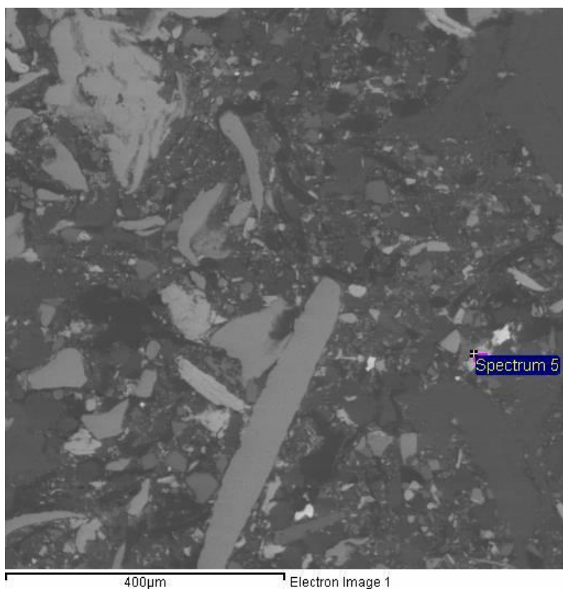
Slika 115. Područje četvrtre analize površine uzorka kočione obloge
