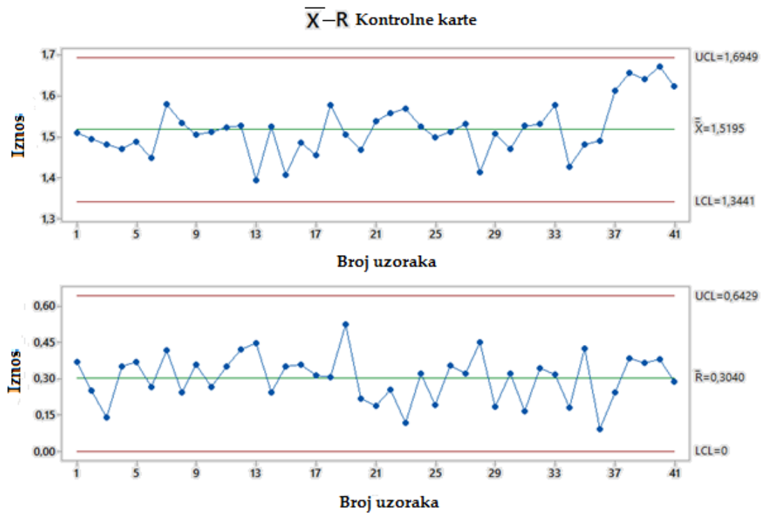
Slika 21. Nove kontrolne karte
