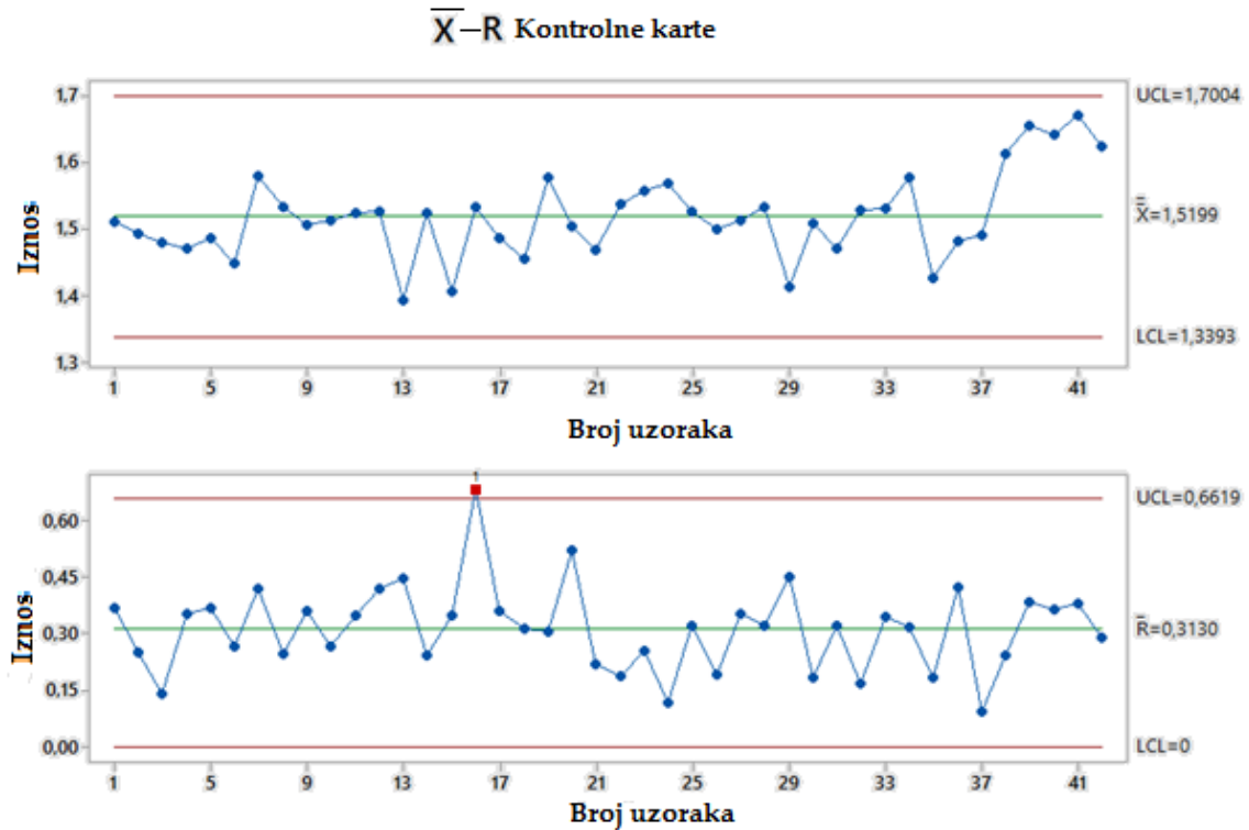
Slika 20. \bar{x}-R kontrolne karte
