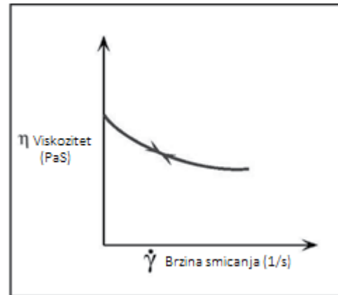
Slika 3.7 Ovisnost prividne viskoznosti o brzini smicanja za nenewtonovsku pseudoplastičnu tekućinu (prema[20])
