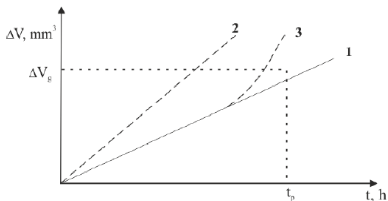
Slika 5.8. Proces trošenja erozijom česticama [4]
