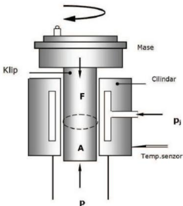
Slika 3: Sklop klip/cilindar
