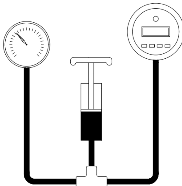
Slika 16: Shematski prikaz mjernje linije
