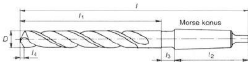
Slika 3. Prikaz dijelova svrdla s koničnom drškom[4]
