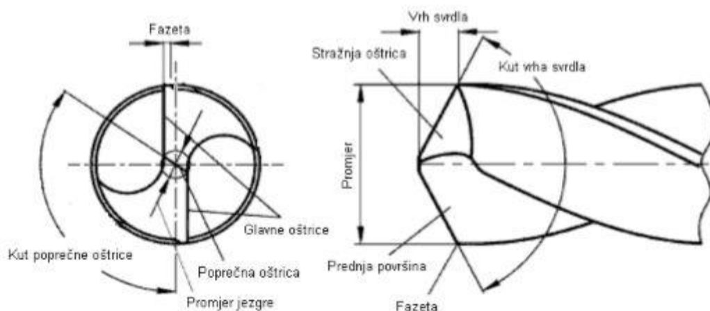
Slika 4. Naziv konstruktivnih elemenata spiralnog svrdla
