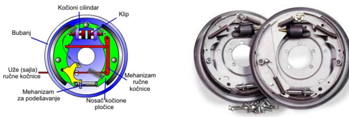
Slika 12. Dijelovi bubanj (čeljusne) kočnice [13]
