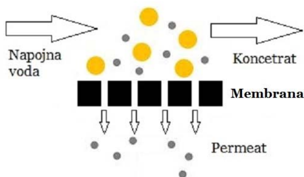
Slika 19. Prikaz tangencijalne filtracije
