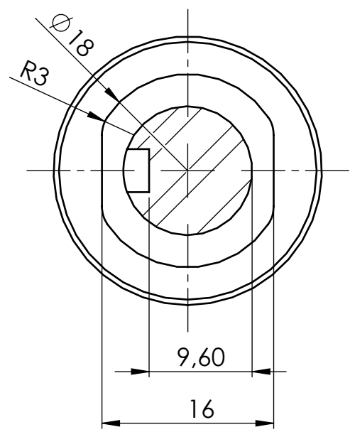
Presjek Y-Y M 2:1
