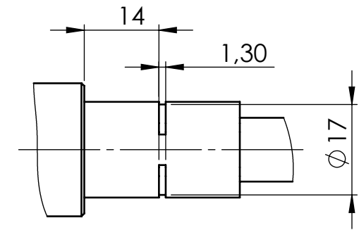
Detalj C M 1:1
