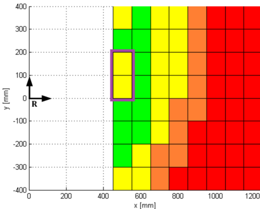
Slika 44 – Područje smanjenih radnih mogućnosti u blizini robota
