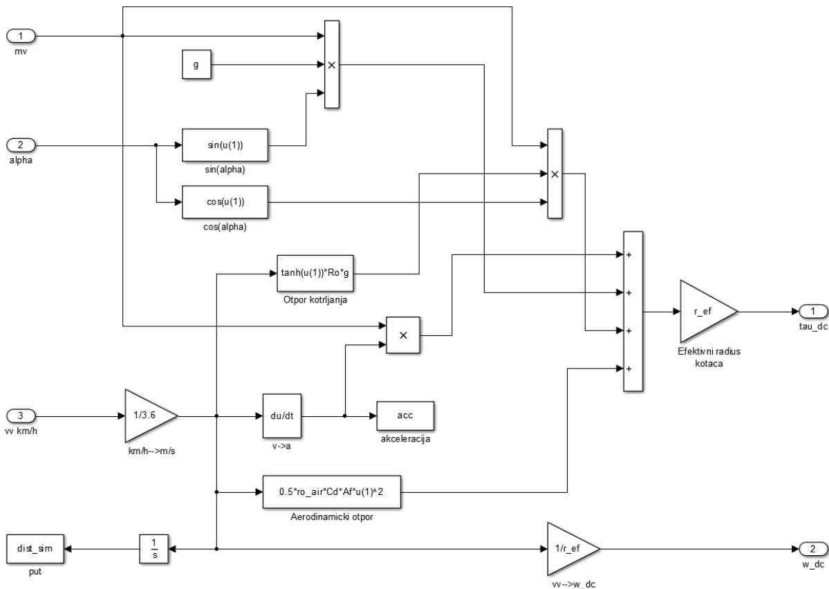
Slika 17: Implementacija jednadžba gibanja u Simulinku
