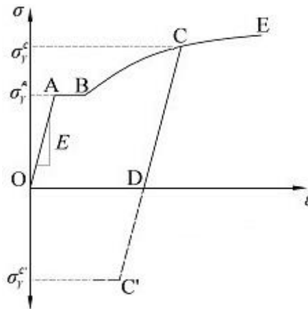
Slika 3.5. Dijagram ovisnosti stvarnog naprežanja o deformaciji
