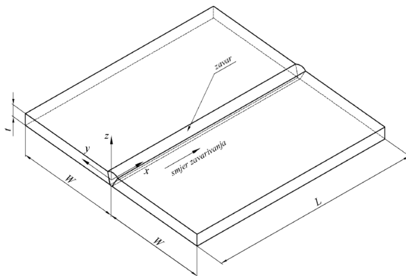
Slika 6.5. Geometrija sučeonog zavarenih ploča
