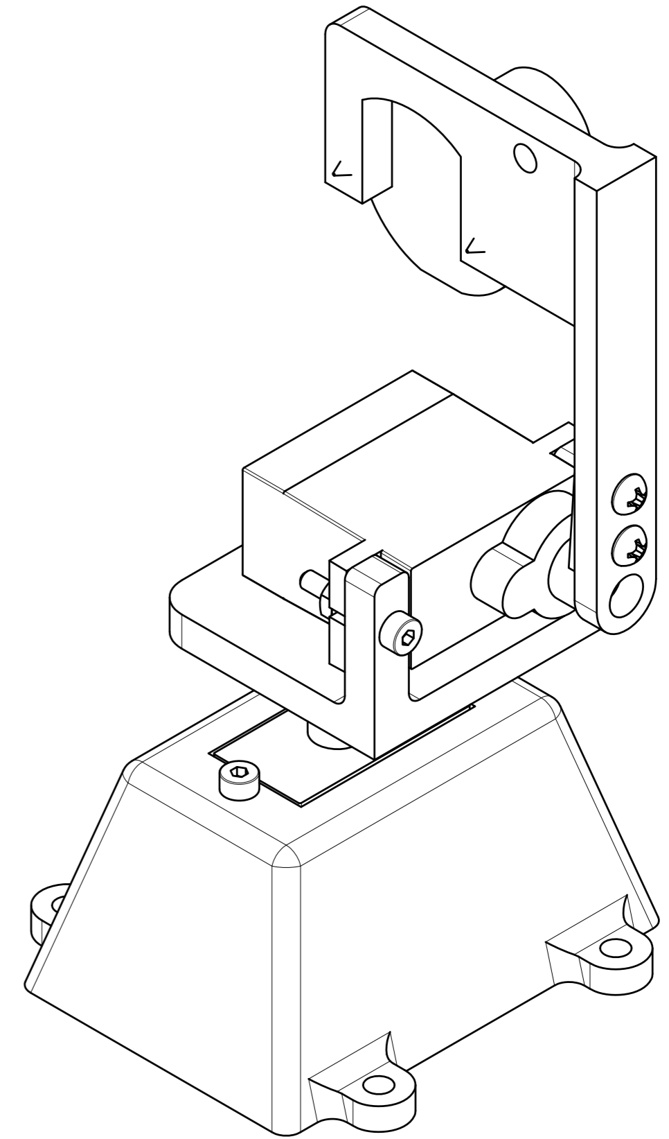
Izometrija M2:1
