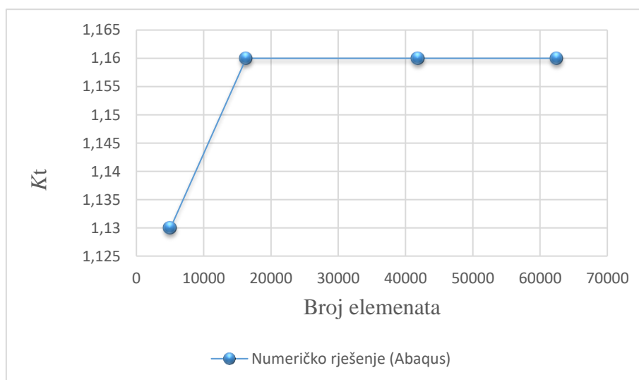
Slika 65. Konvergencija faktora koncentracije naprezanja za konzolu s promjenjivim poprečnim presjekom i eliptičnim zaobljenjem
