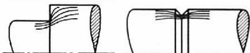
Slika 10. Mjesta koncentracije naprezanja kod vratila
