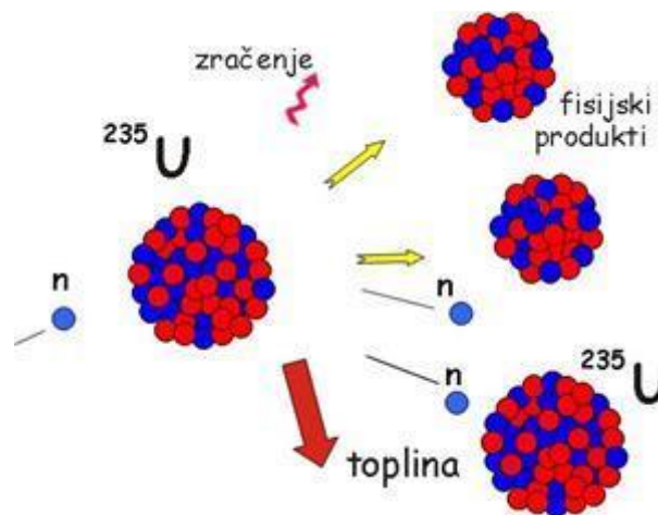
Slika 1.1 Postupak fisije
