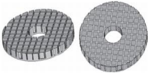
b) 1-3 piezoelektrični kompozit.
