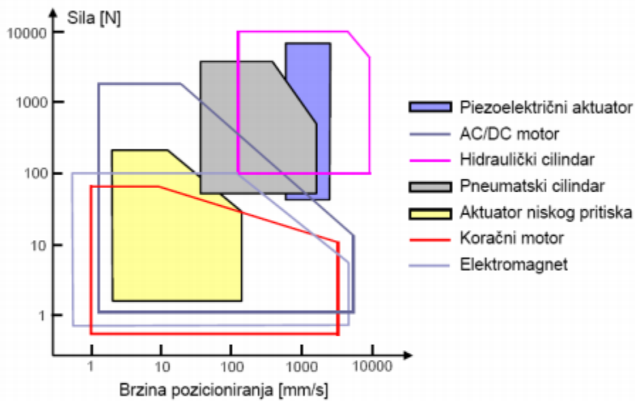
Slika 24: Ovisnost sile o brzini pozicioniranja [11]
