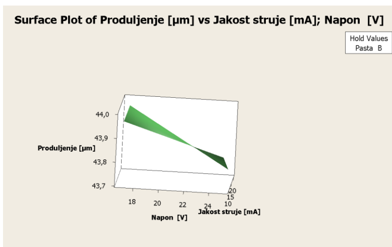
Slika 57: Graf odzivne površine za pastu B (2)
