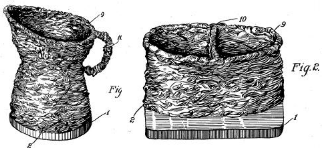
Slika 5: Proizvodi dobiveni nizanjem sloj po sloj [9]
