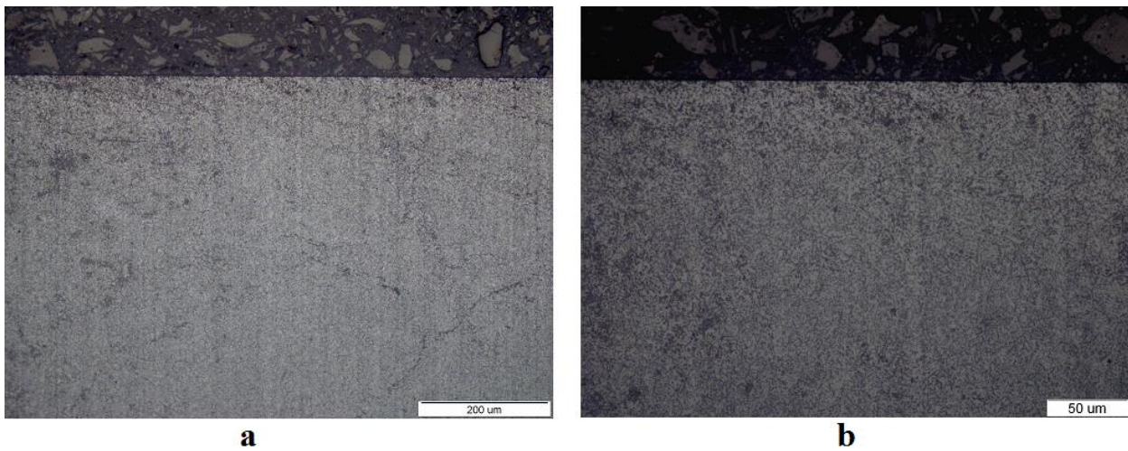
Slika 60. Mikrostruktura rubnog sloja uzorka D2: a) 200x, b) 500x
