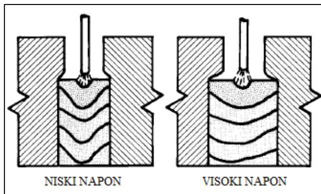
Slika 13. Utjecaj napona zavarivanja na izgled taline [1]
