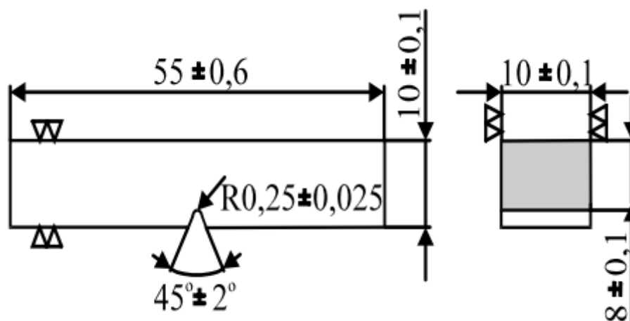
Slika 42. Oblik i dimenzije epruvete s V utorom za ispitivanje udarne radnje loma [24]
