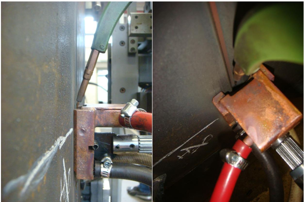
Slika 27. Položaj elektrode prije zavarivanja
